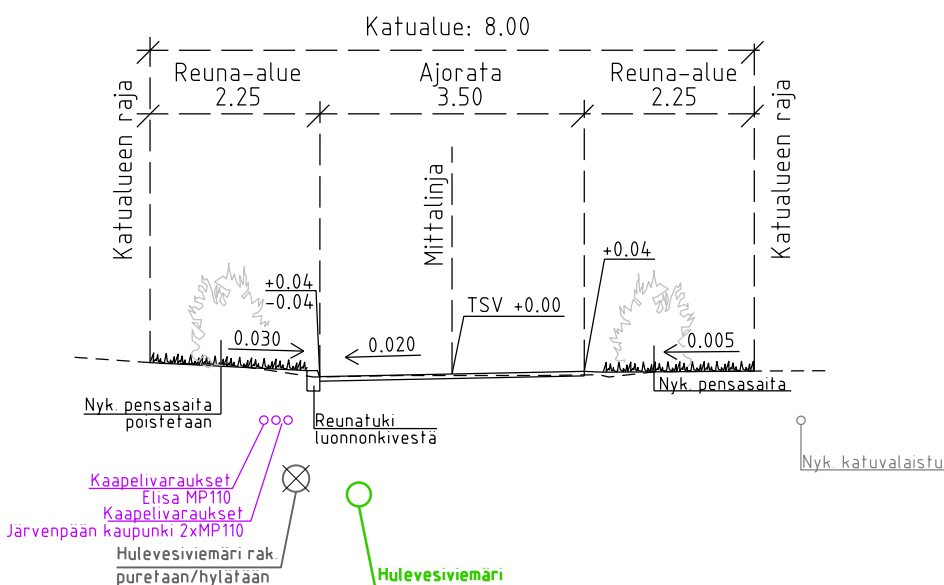
Mesiheinänkuja Tyyppipoikkileikkaus plv 31-90 (pl 55) 1:100
