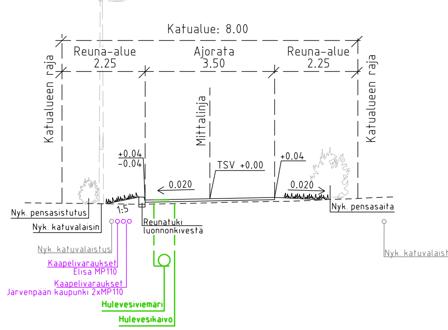
Mesiheinänkuja Tyyppipoikkileikkaus plv 5-25, 95-118 (pl 110) 1:100
